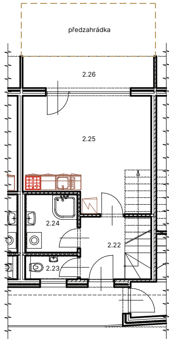
PŮDORYS 2.NP
