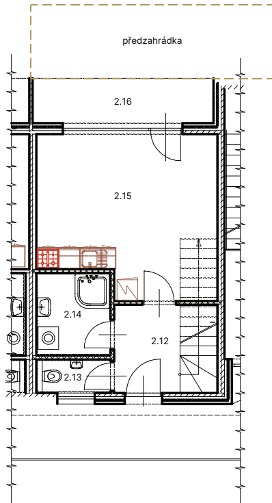
PŮDORYS 2.NP
