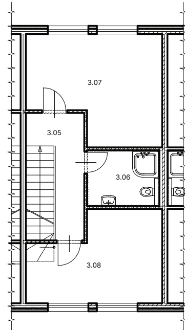
PŮDORYS 3.NP
