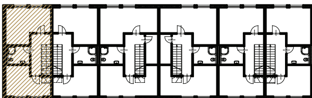
PŮDORYS 3.NP
